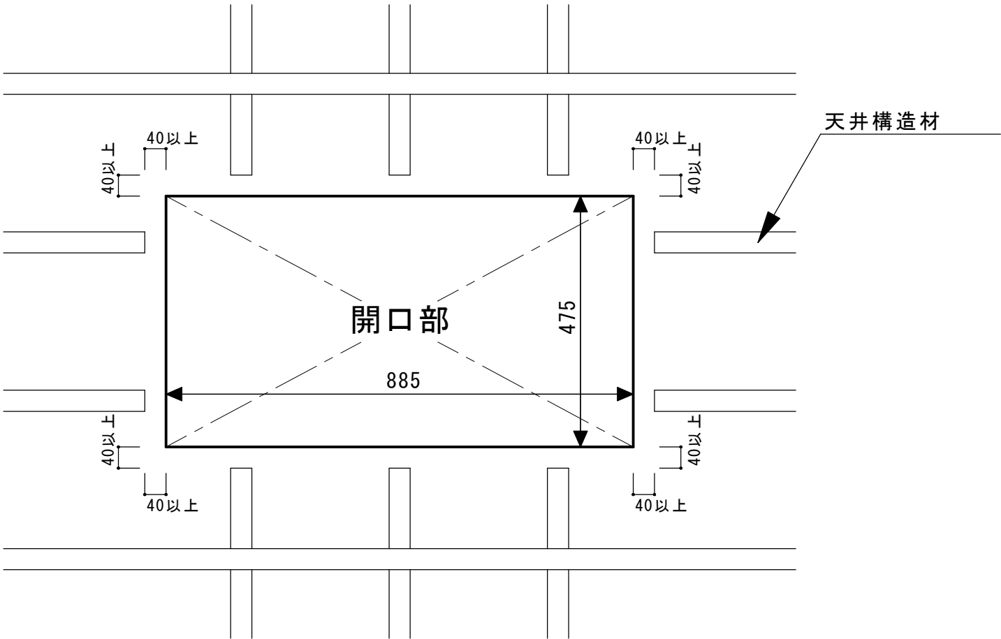
【天井裏平面図】
