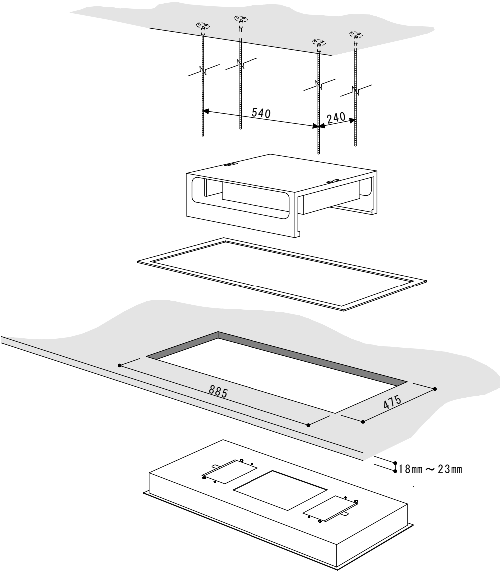
【天井開口寸法】
