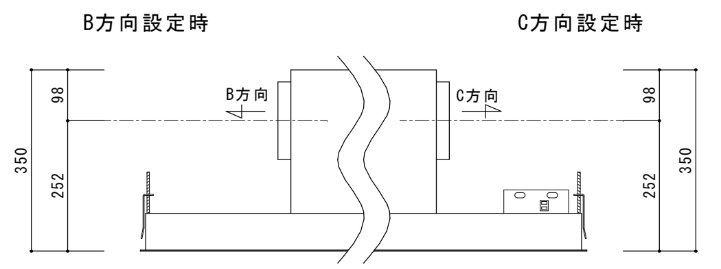
【排気方向変更時寸法】
