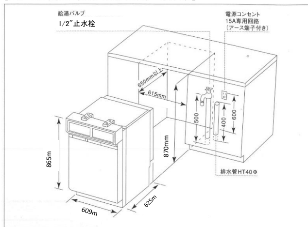
[ユニット開口寸法と設備例(一次側)]
